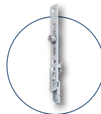
Terminal con cierre de rodillo 150 mm, para presión adicional de contacto Art. no. 91DXVR150R
