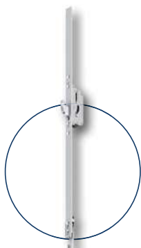
Extensión con cierre de gancho 740 mm, cierre adicional superior para puertas muy altas Art. no. 91MAO607406X
