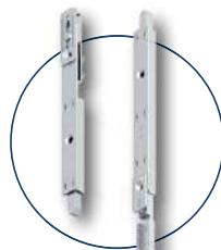
Terminal de cierre 150 mm, para seguridad extra y mayor presión de contacto ideal para puertas de dos hojas Superior - Art. no. 91MV150186S Inferior - Art. no. 91MV15018B6S
