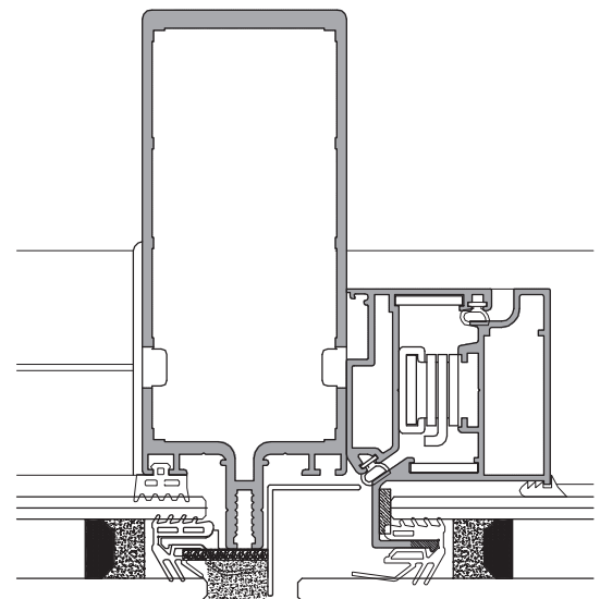
SISTEMA ESTRUCTURAL DIRECTO
